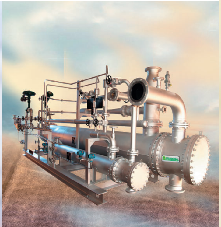
PRESION DE ASPIRACION: 75 TORR DISEÑADO PARA LA ELIMINACION DEL AGUA DEL DIESEL
