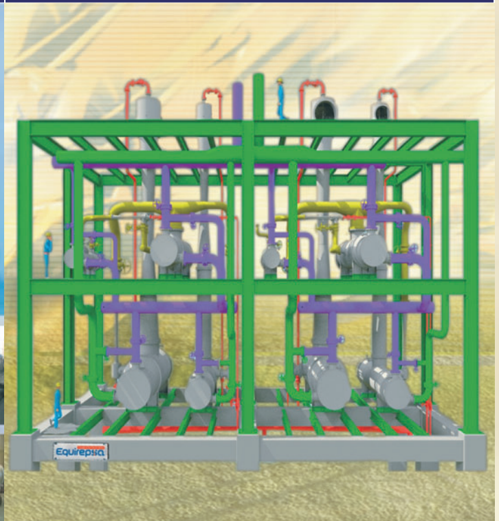
PRESION DE ASPIRACION: 8.5 TORR DISEÑADO PARA LA PRODUCCION DE VACÍO EN COLUMNA PREPARATORA DE CARGA EN LA LINEA DE REFINACION DE CRUDO DE PETROLEO
