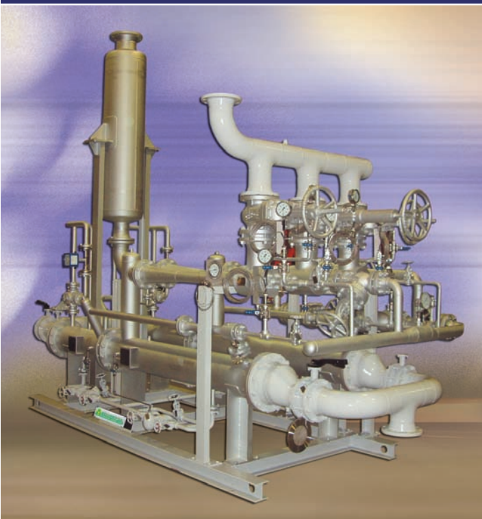
PRESION DE ASPIRACION: 24TORR. EXTRACCION A VACÍO DE UNA MEZCLA DE AIRE Y VAPOR EN UN CONDENSADOR
