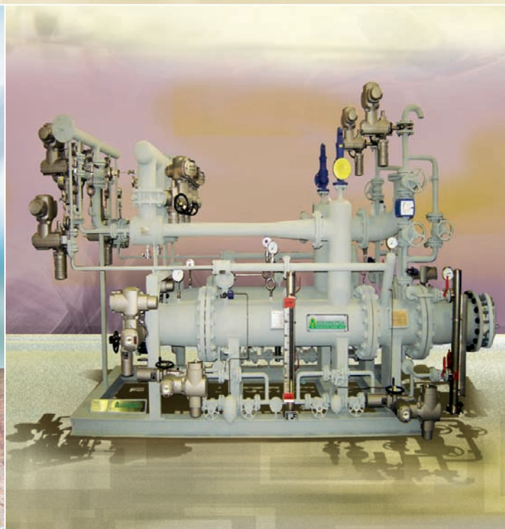
PRESION DE ASPIRACION: 67 TORR. EXTRACCION A VACIO DE UNA MEZCLA DE AIRE/ VAPOR SATURADO EN UN CONDENSADOR
