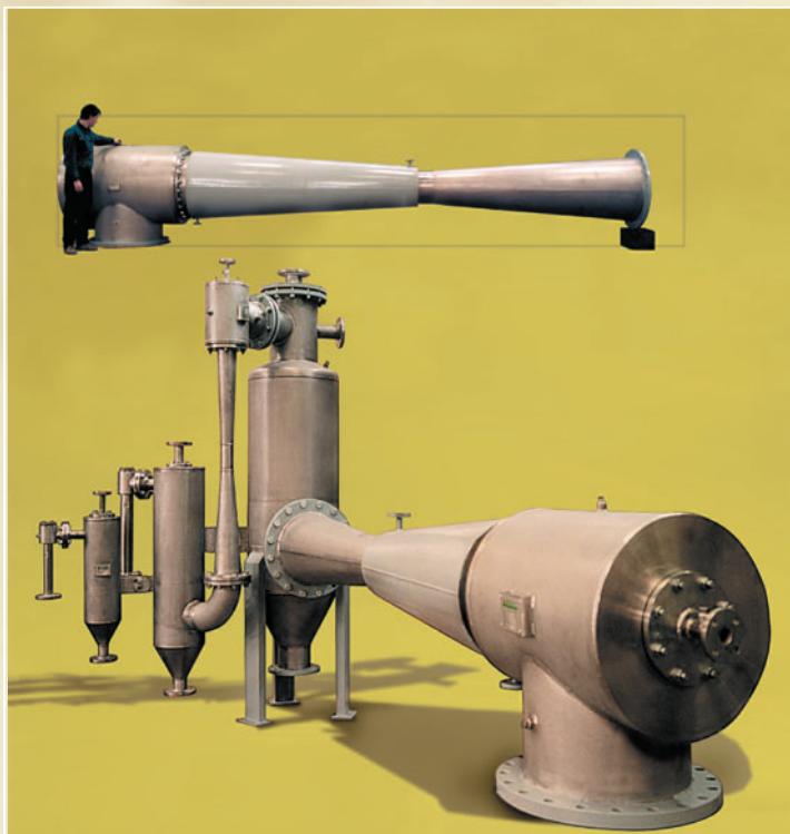
PRESION DE ASPIRACION: 1 TORR A. AGUA HELADA 6,5 °C DISEÑADO PARA LA DESODORIZACION DE ACEITE COMESTIBLE
