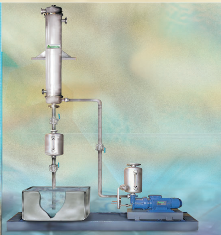
PRESION DE ASPIRACION: 67 TORR. DISEÑADO PARA LA PRODUCCION DE VACIO EN UNA PLANTA DE FRUTOS SECOS
