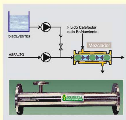
MEZCLADORES ESTÁTICOS STATIC MIXERS
