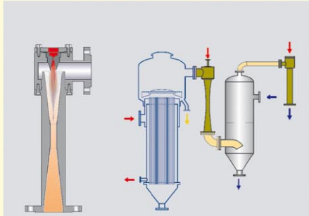
EYECTORES / EJECTORS
