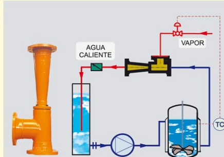
CALENTADORES / HEATERS
