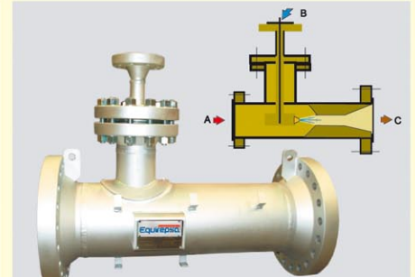
ATEMPERADOR / DESUPERHEATER
