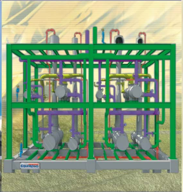
PRESION DE ASPIRACION: 8.5 TORR DISEÑO PARA LA PRODUCCION DE VACÍO EN COLUMNA PREPARADORA DE CARGA EN LA LINEA DE REFINACION DE CRUDO DE PETROLEO
